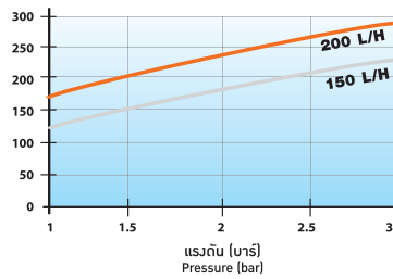
อัตราการจ่ายน้ำ (ลิตร/ชม.) Flow rate (L/H)
