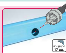
เจาะท่อพีวีซี ด้วยดอกสว่านขนาด 17 มม.
