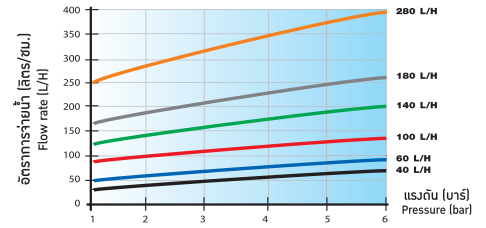
ตารางแสดงอัตราการจ่ายน้ำ รุ่น WING-S
