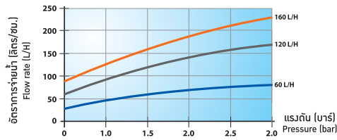
ตารางแสดงอัตราการจ่ายน้ำ รุ่น WING-F4
