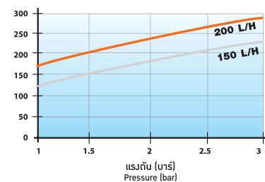
อัตราการจ่ายน้ำ (ลิตร/ชม.) Flow rate (L/H)
