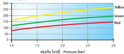
อัตราการจ่ายน้ำ (ลิตร/ชม.) Flow rate (L/H)
