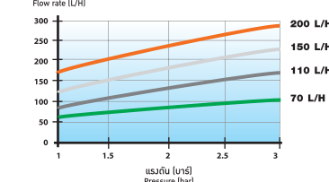
อัตราการจ่ายน้ำ (ลิตร/ชม.) Flow rate (L/H)
