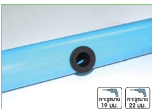
เจาะรูท่อพีวีซี ขนาด 19 มม. (ลูกยาง GR 20) เจาะรูท่อพีวีซี ขนาด 22 มม. (ลูกยาง GR 25)
