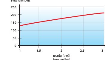
อัตราการจ่ายน้ำ (ลิตร/ชม.) Flow rate (L/H)
