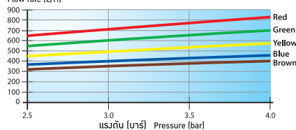
อัตราการจ่ายน้ำ (ลิตร/ชม.) Flow rate (L/H)
